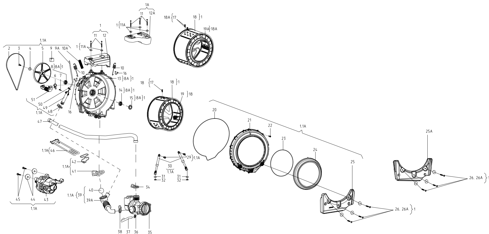
Рисунок 4 - Колебательная система
