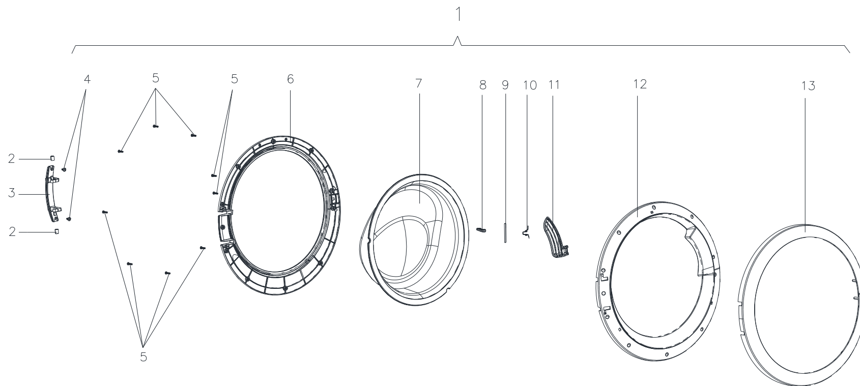
Рисунок 5 - Дверца
