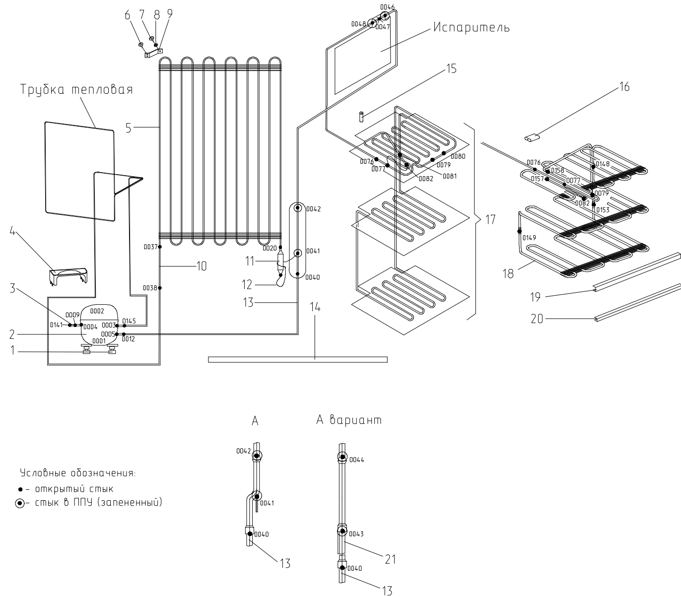
Рисунок 4 - Схема холодильного агрегата
