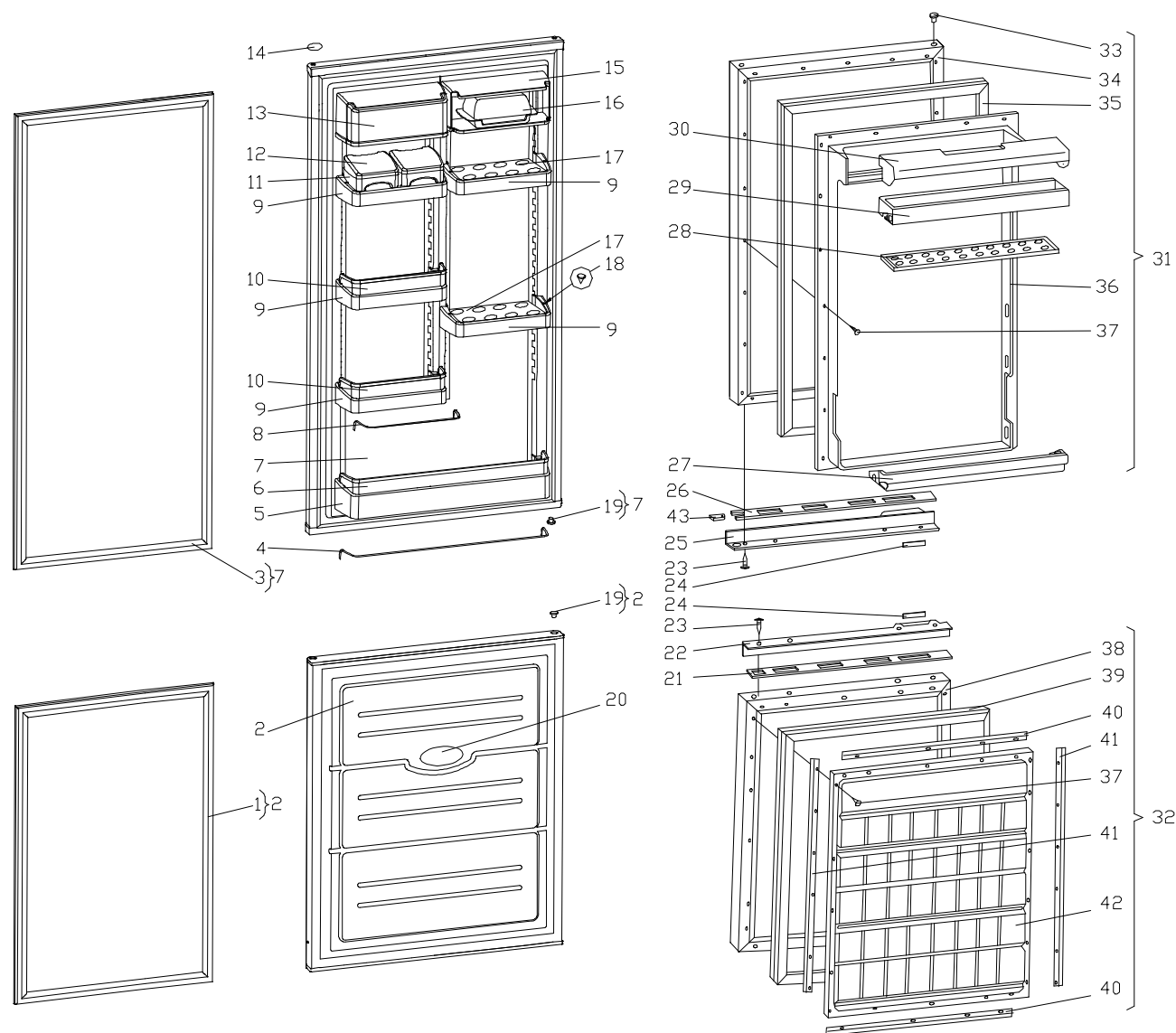
Рисунок 3 - Двери
