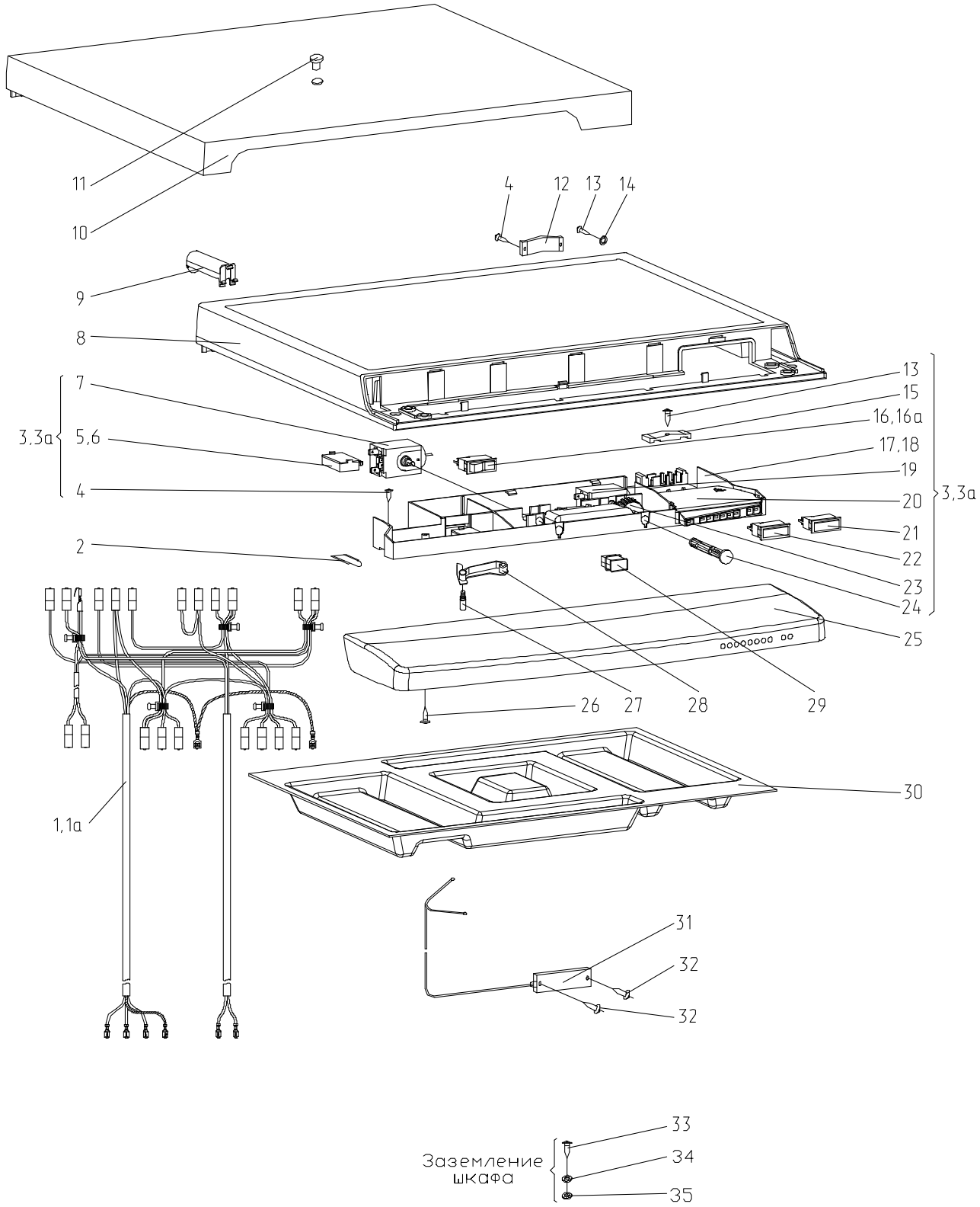
Рисунок 5 - Электропроводка
