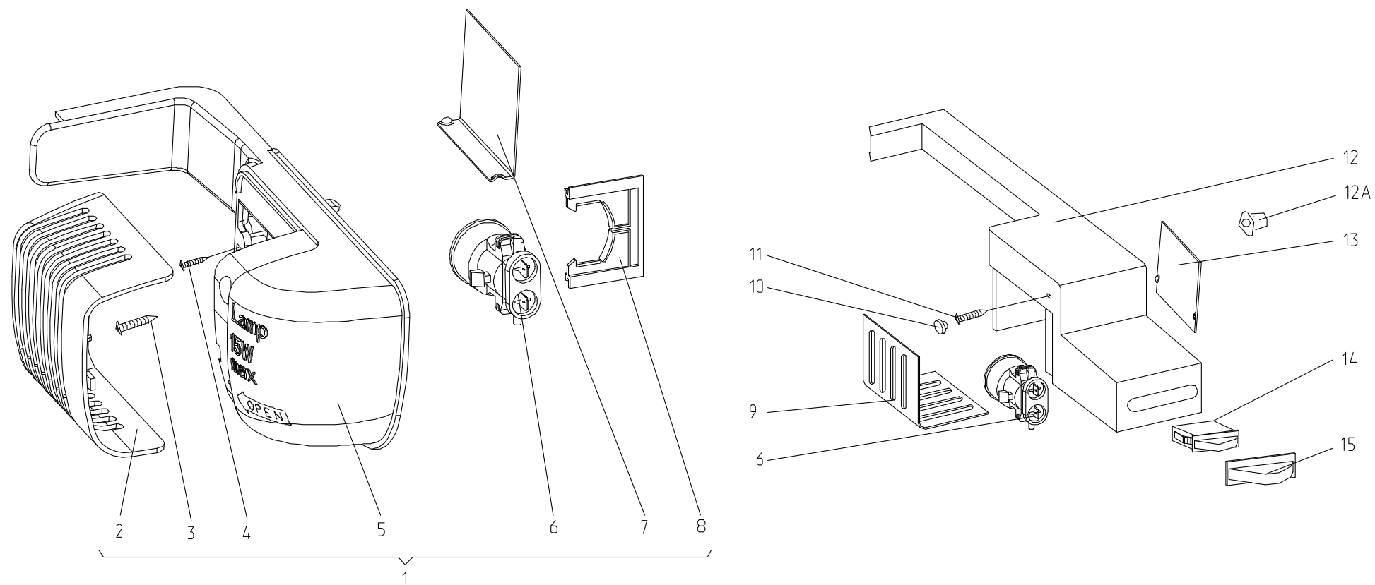
Рисунок 6 - Панель монтажная
