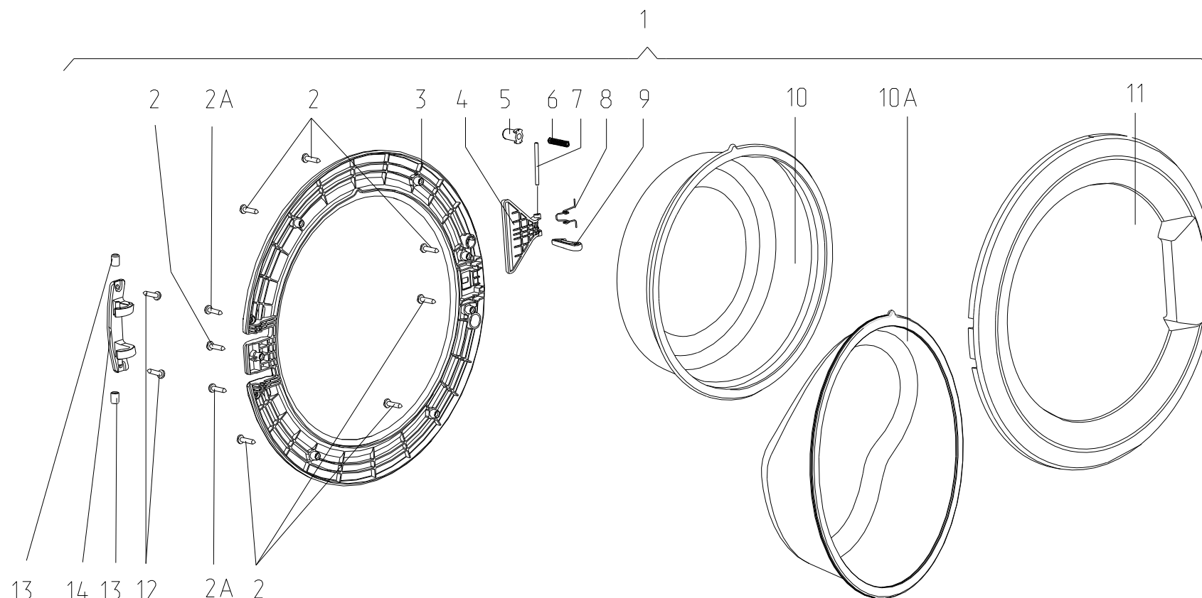
Рисунок 4 - Дверца
