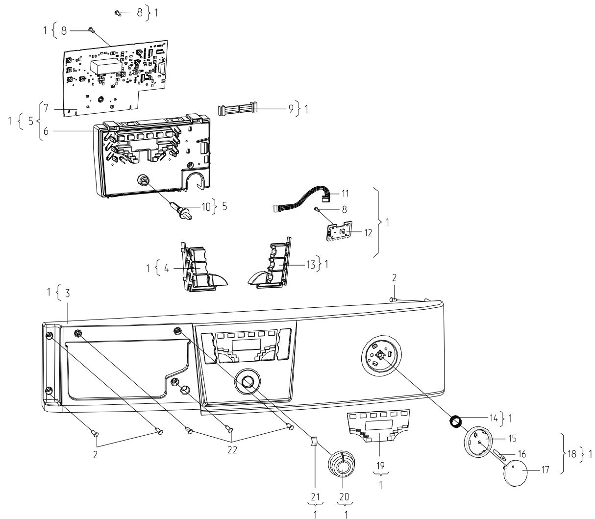
Рисунок 2 - Панель управления
