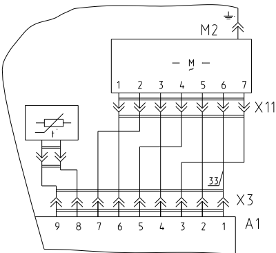
Рисунок А.2 - Схема электрическая принципиальная Остальное см. рисунок А.1
