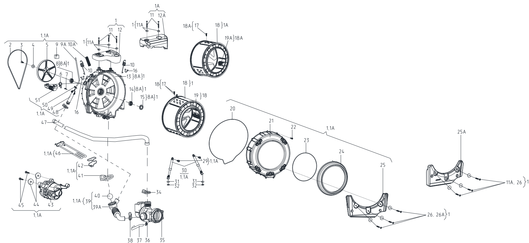
Рисунок 4 - Колебательная система
