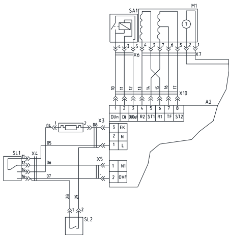
Рисунок А.4- Схема электрическая принципиальная и соединений СМА 60Y1210-A-XX, СМА 70C1410-A-XX Остальное см. рис. 1
