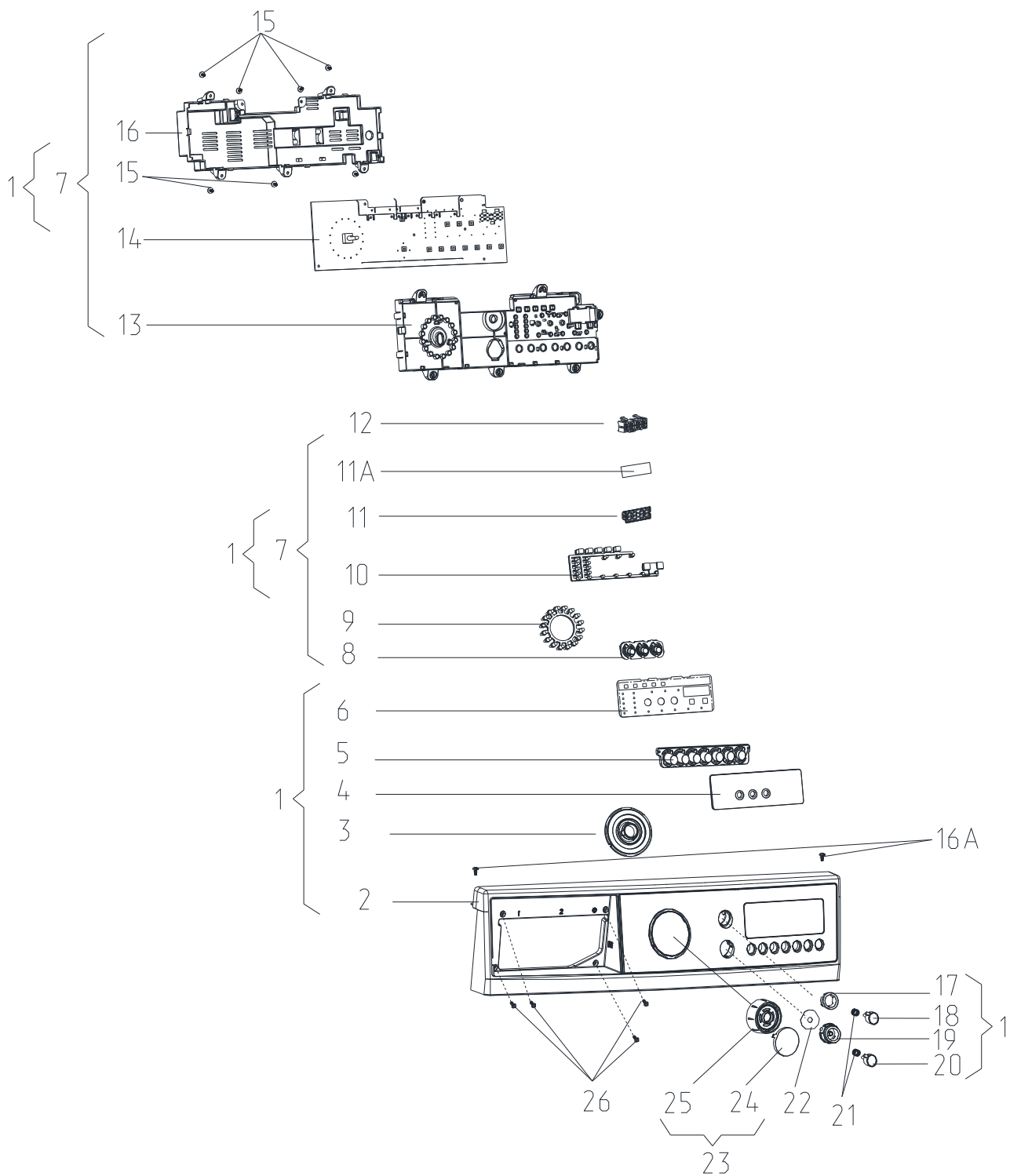
Рисунок 2 - Панель управления
