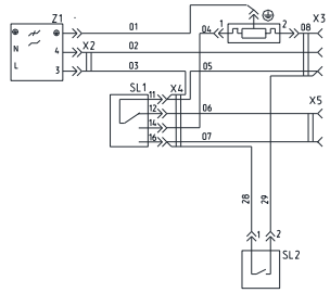
Рисунок А.2- Схема электрическая принципиальная и соединений СМА 70C1210-A-XX Остальное см. рис. 1
