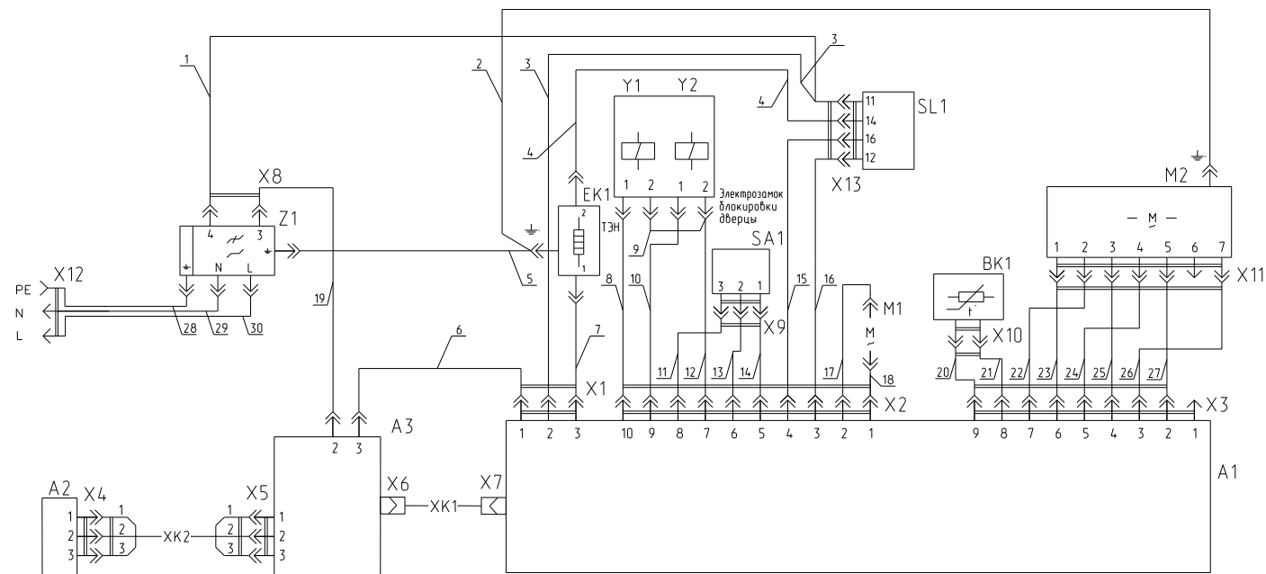
Рисунок А.1 - Схема электрическая принципиальная и соединений
