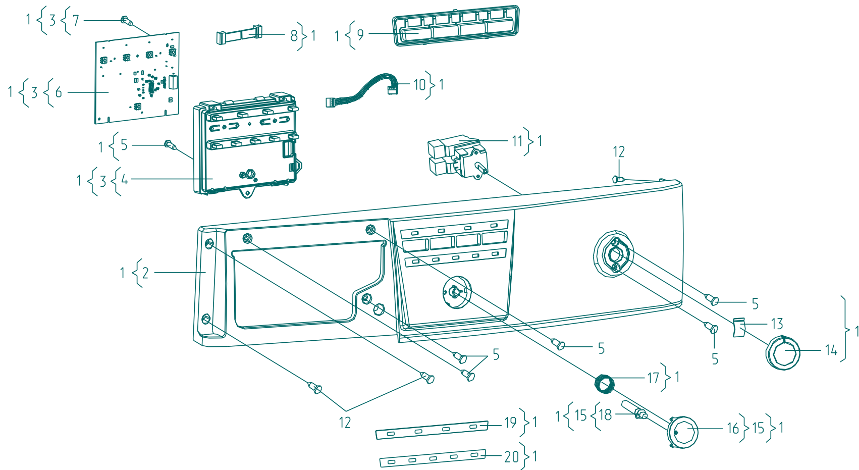
Рисунок 2 - Панель управления
