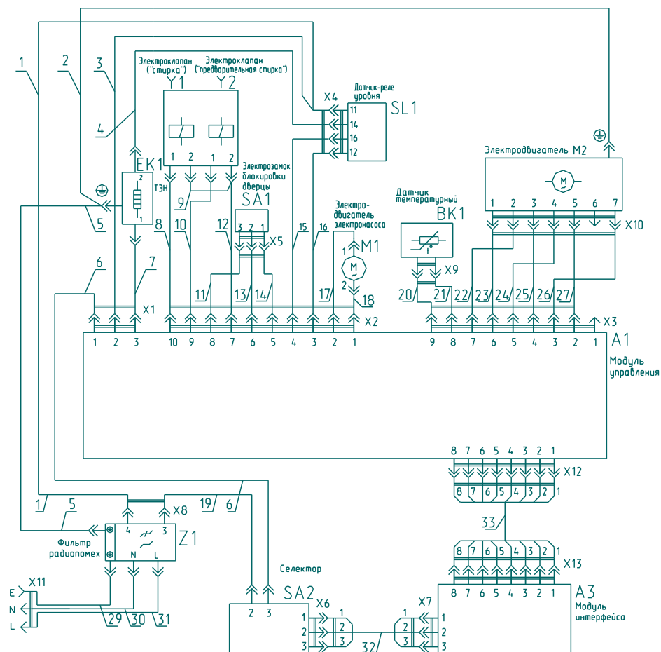
Рисунок А.1 - Схема электрическая принципиальная и соединений машин СМА 35М101-XXX, СМА 35М81-XXX, СМА 45У101-XXX, СМА 45У81-XXX, СМА 50С101-XXX, СМА 50С121-XXX, СМА 50С81-XXX, СМА 60К81-XXX, СМА 60К101-XXX
