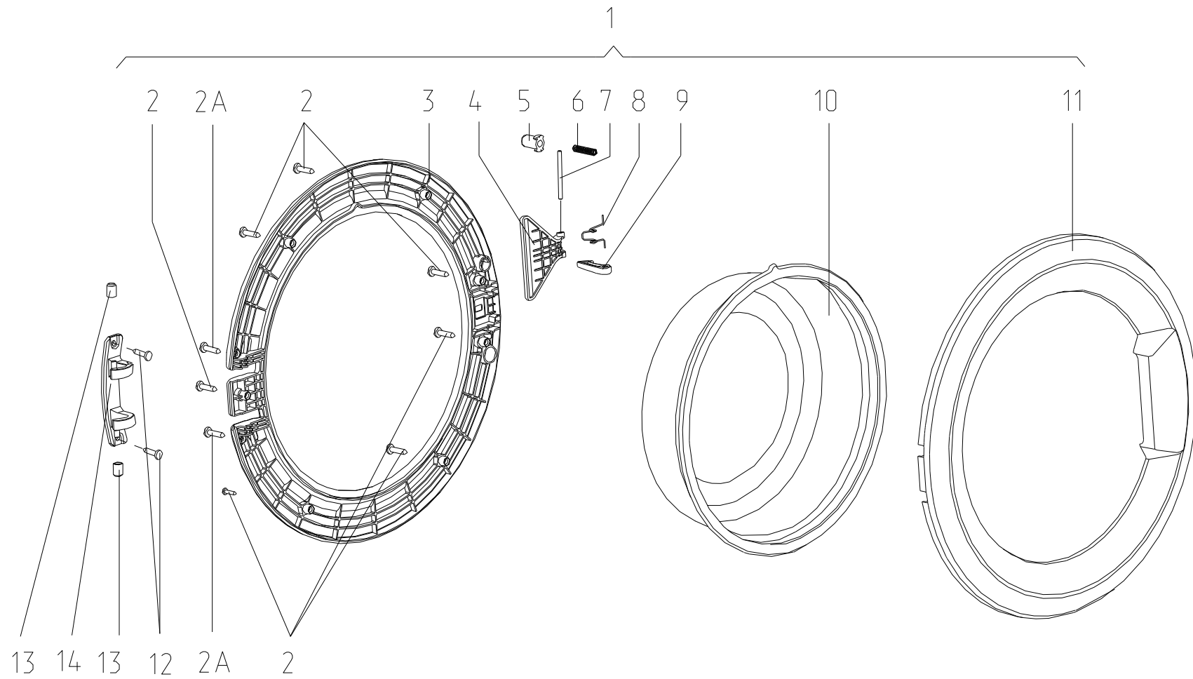
Рисунок 5 - Дверца
