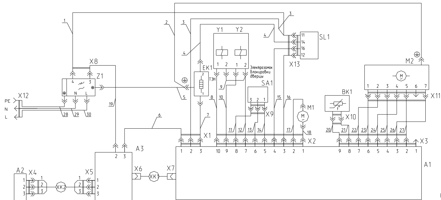
Рисунок А.3 - Схема электрическая принципиальная и соединений машины СМА 40М102-ХХ
