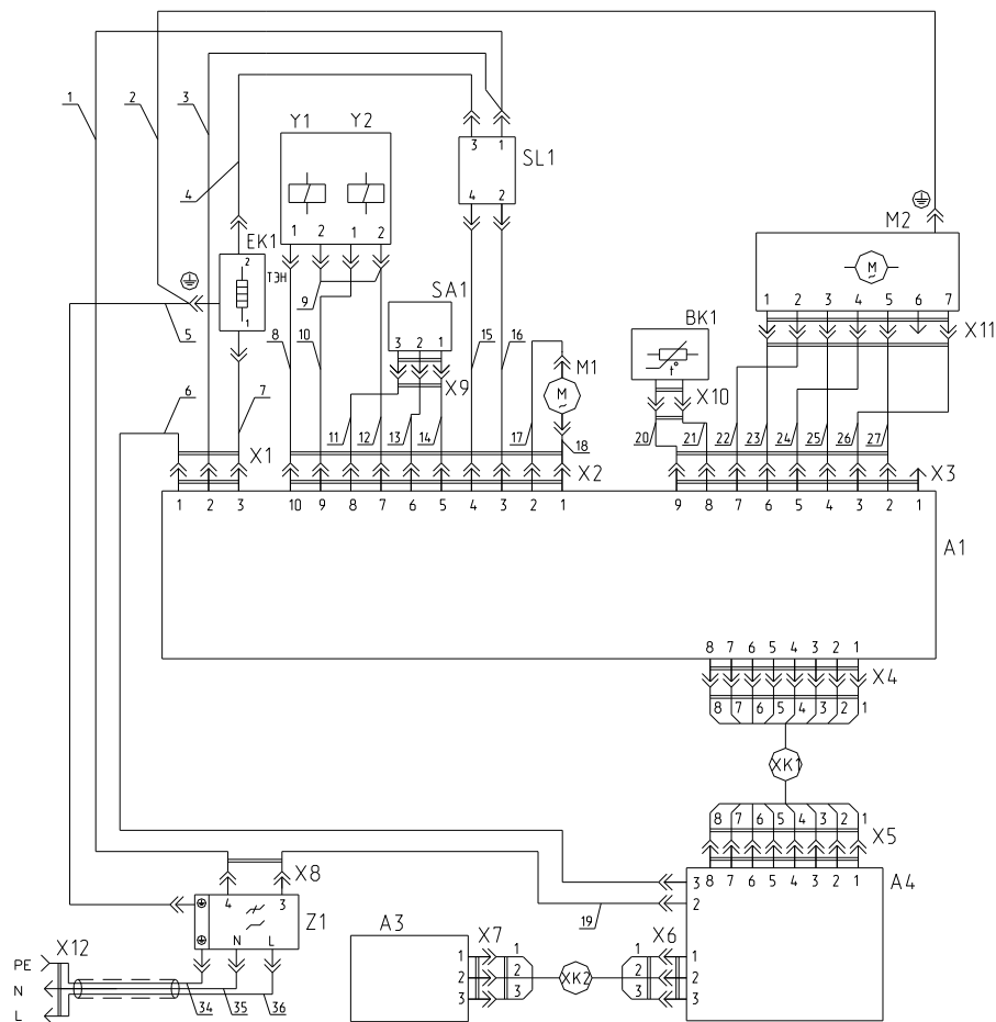
Рисунок А.1 – Схема электрическая принципиальная и соединений машин СМА 50С82-000, СМА 35М102-000, СМА 45У102-000
