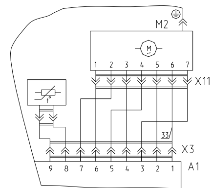
Рисунок А.4 - Схема электрическая принципиальная и соединений машины СМА 40М102-ХХ Остальное см. рисунок А.3
