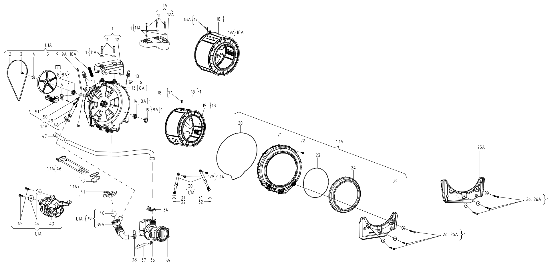
Рисунок 4 - Колебательная система
