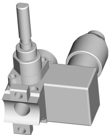
Кран газовый
