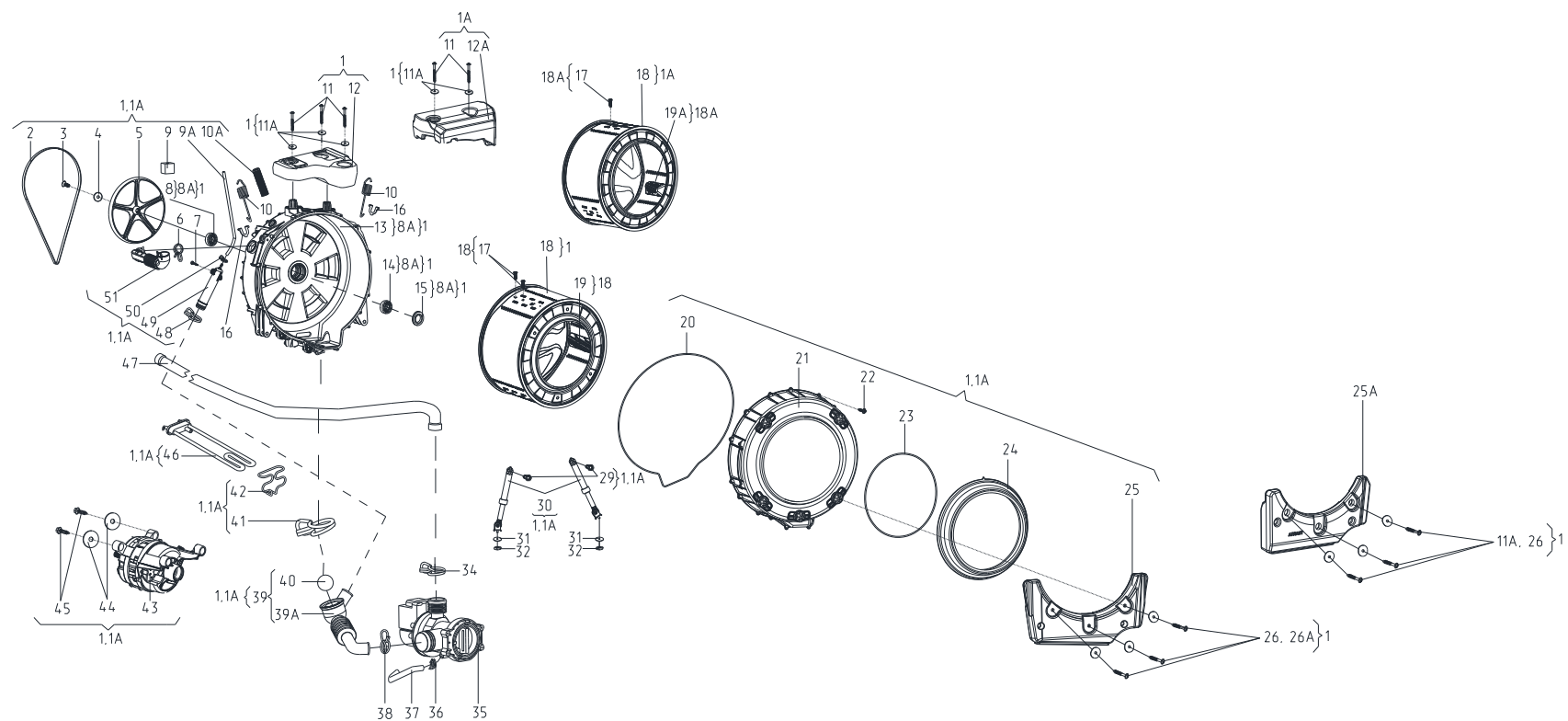
Рисунок 4 - Колебательная система
