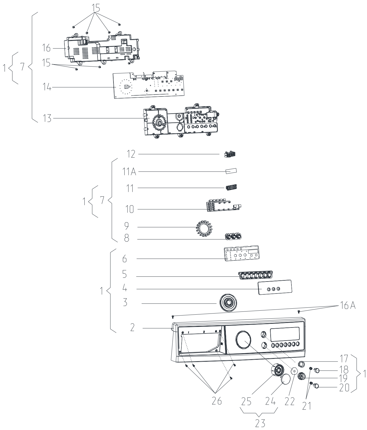
Рисунок 2 - Панель управления
