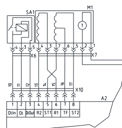
Рисунок А.3- Схема электрическая принципиальная и соединений СМА 60Y1210-XX, СМА 70C1410-XX Остальное см. рис. 1
