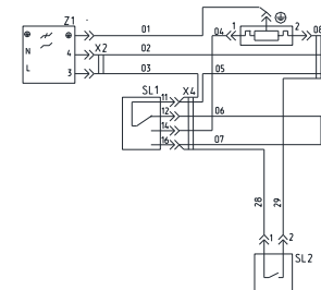
Рисунок А.2- Схема электрическая принципиальная и соединений СМА 70C1210-A-XX
