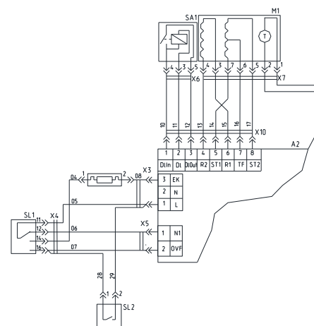
Рисунок А.4- Схема электрическая принципиальная и соединений СМА 60Y1210-A-XX, СМА 70C1410-A-XX
