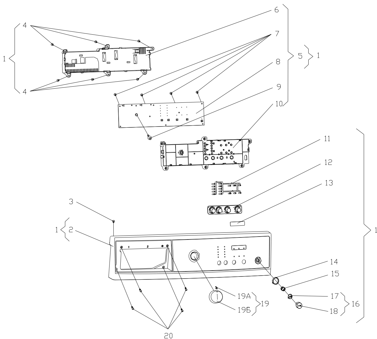
Рисунок 2 - Панель управления
