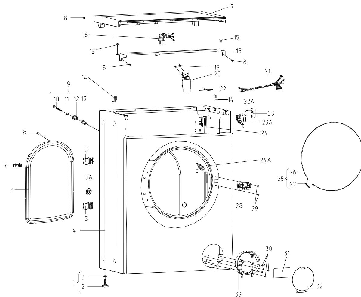
Рисунок 1 - Корпус
