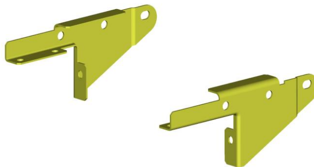
17 Кронштейн стола 6140.00.0.010, -01, -04, -05
