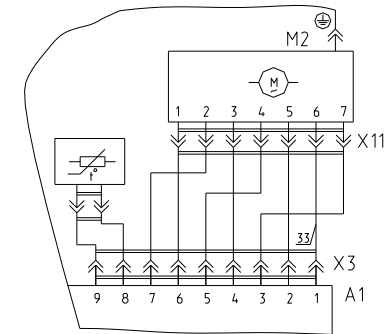
Рисунок А.4 - Схема электрическая принципиальная и соединений машины СМА 40М102-XX Остальное см. рисунок А.3
