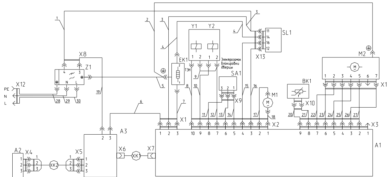
Рисунок А.3 - Схема электрическая принципиальная и соединений машины СМА 40М102-XX
