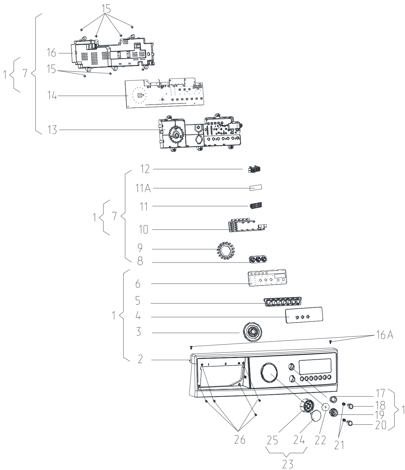
Рисунок 2 - Панель управления
