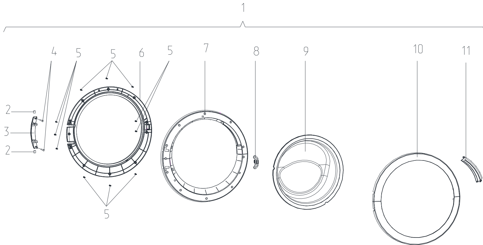
Рисунок 5 - Дверца
