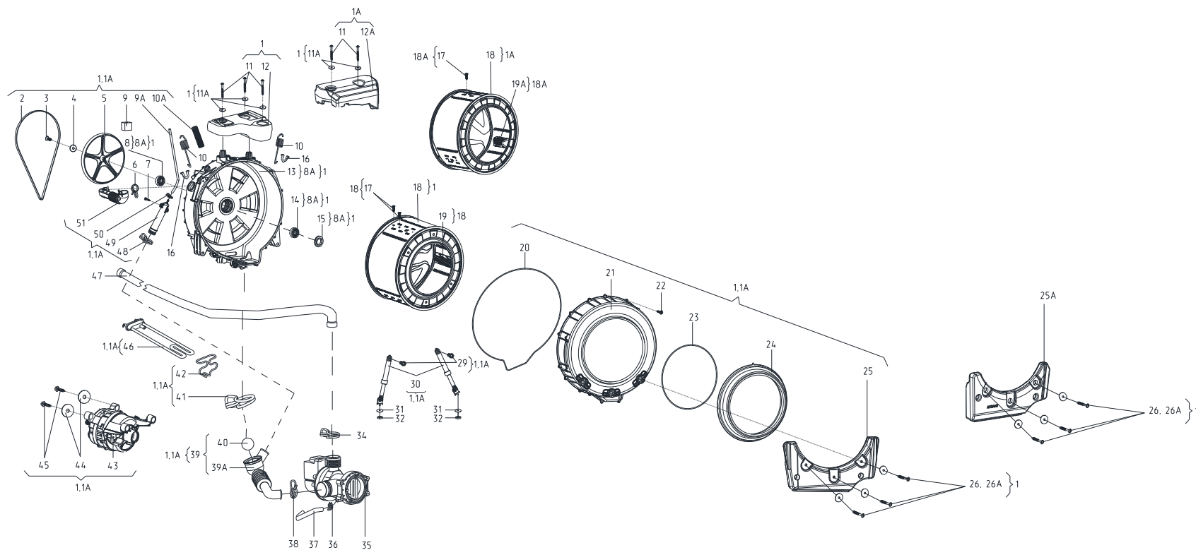
Рисунок 4 - Колебательная система
