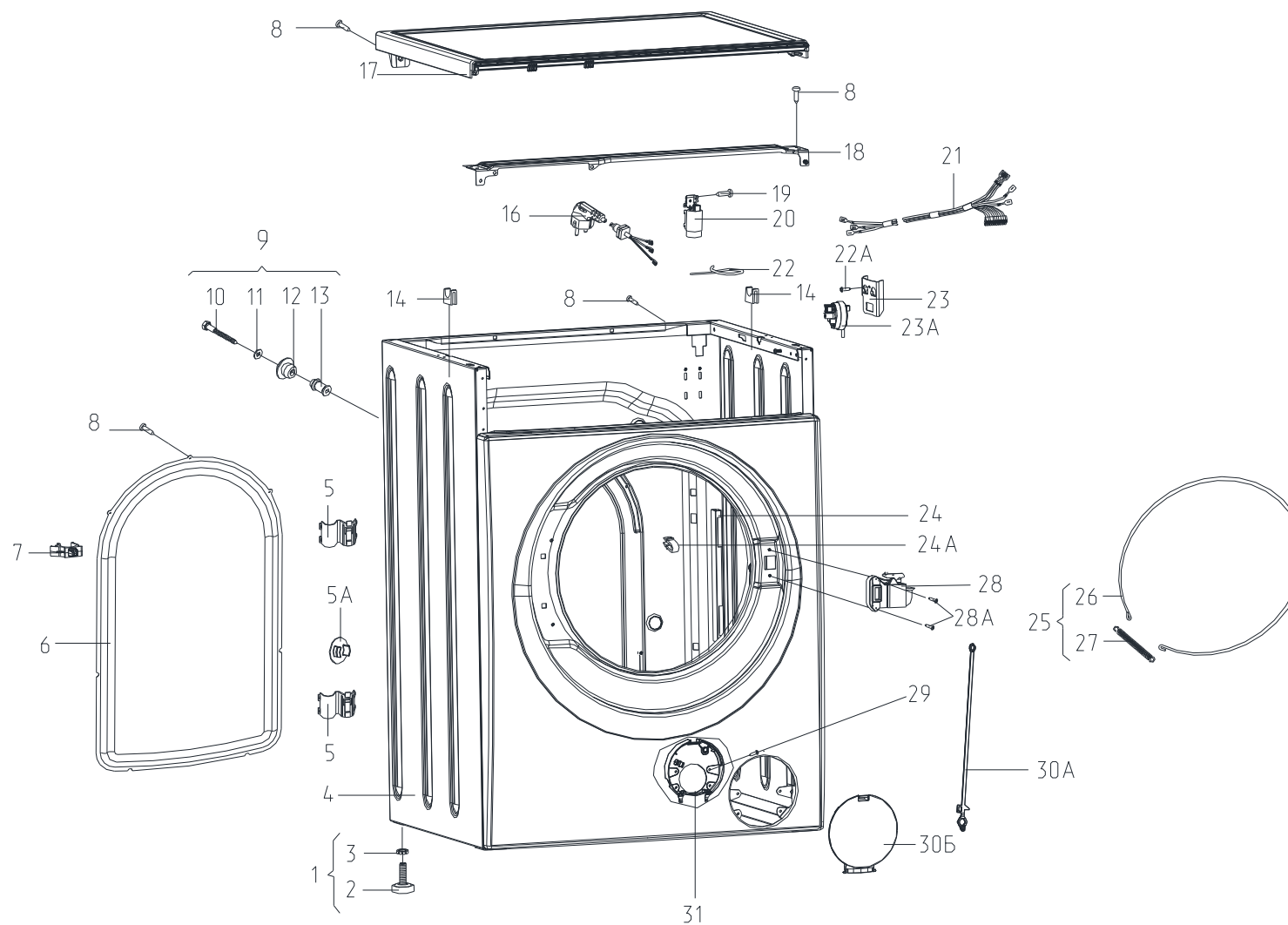
Рисунок 1 - Корпус
