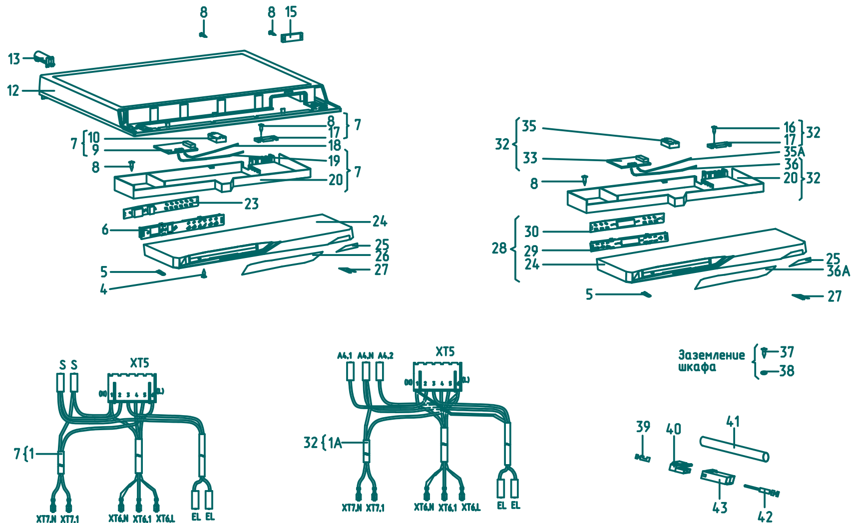
Рисунок 7 - Электропроводка
