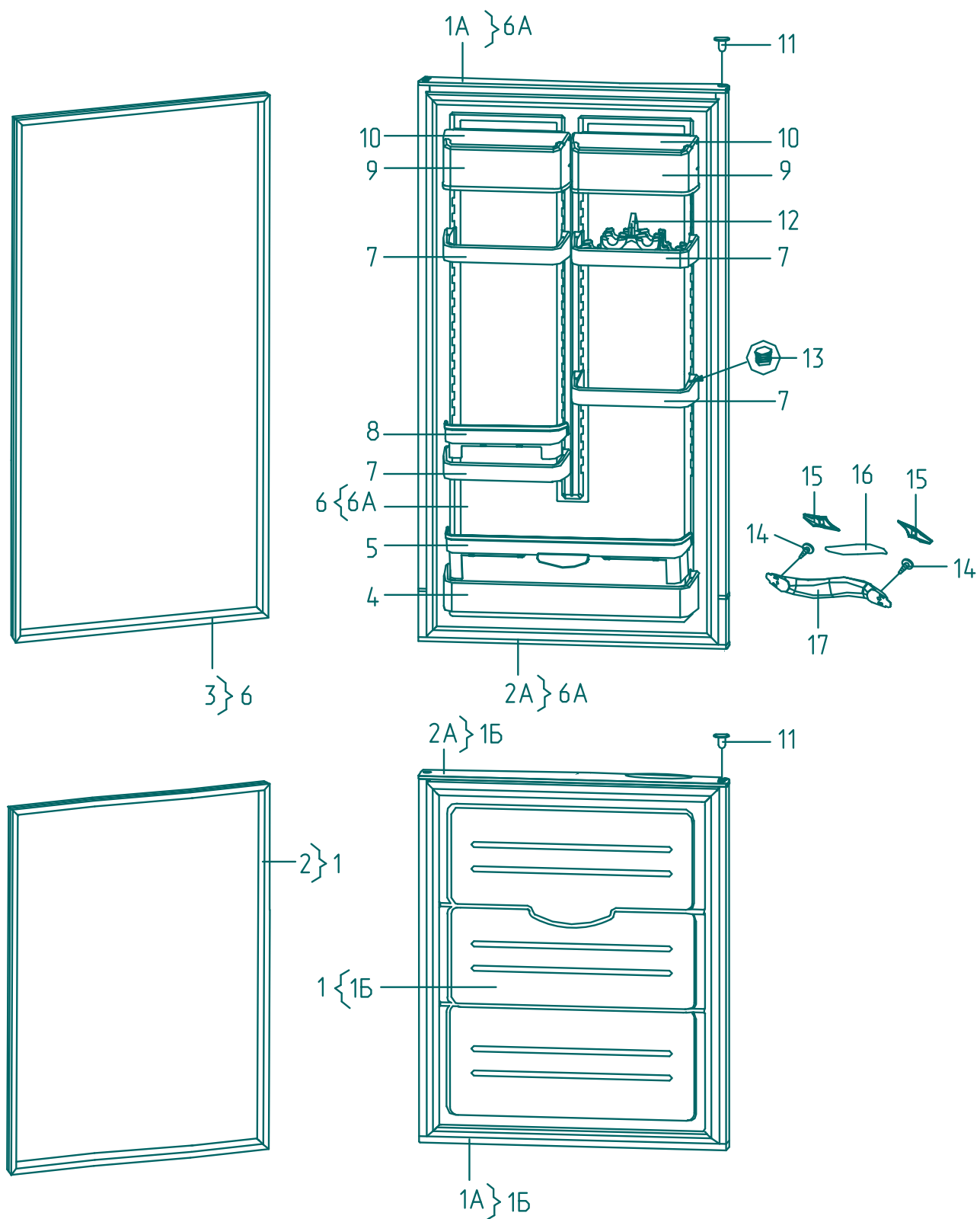
Рисунок 4 - Двери
