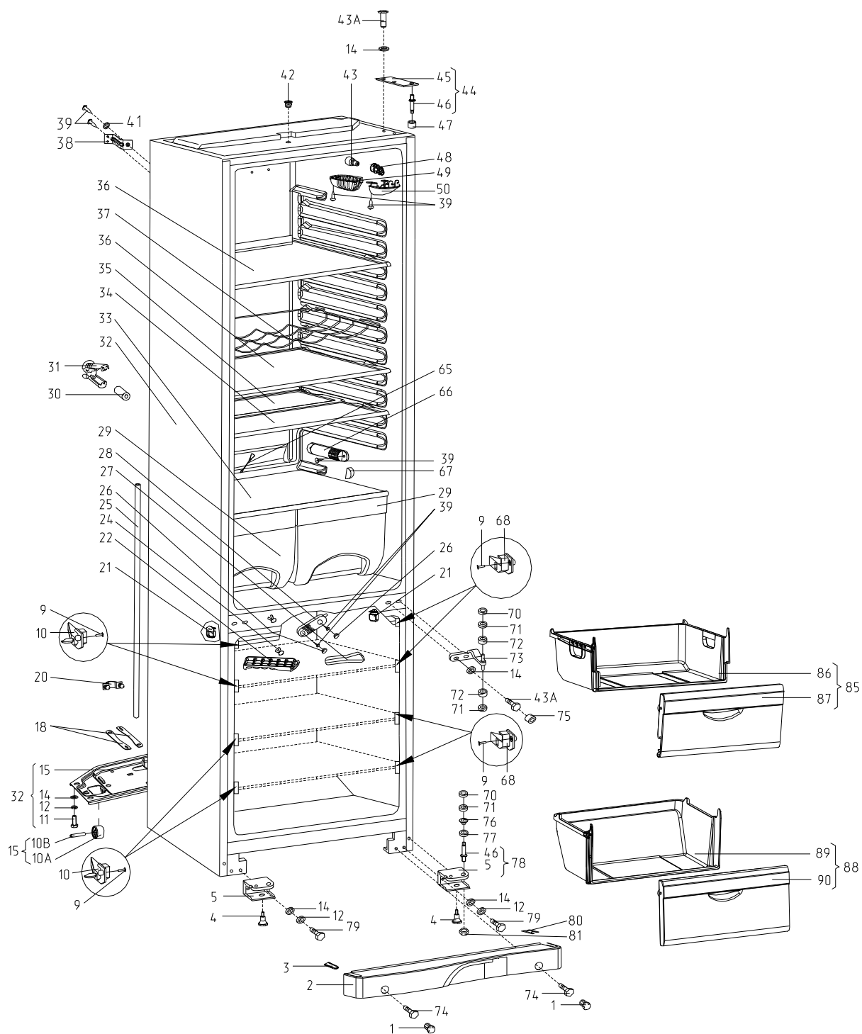
Рисунок 3 - Шкаф
