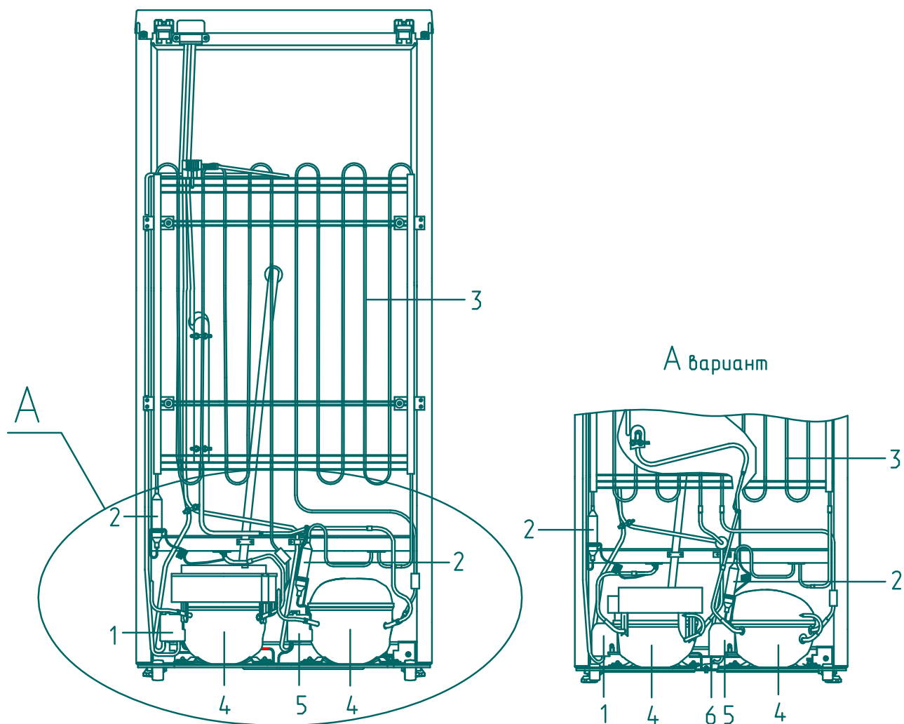
Холодильник с компрессором типа С-КН.
