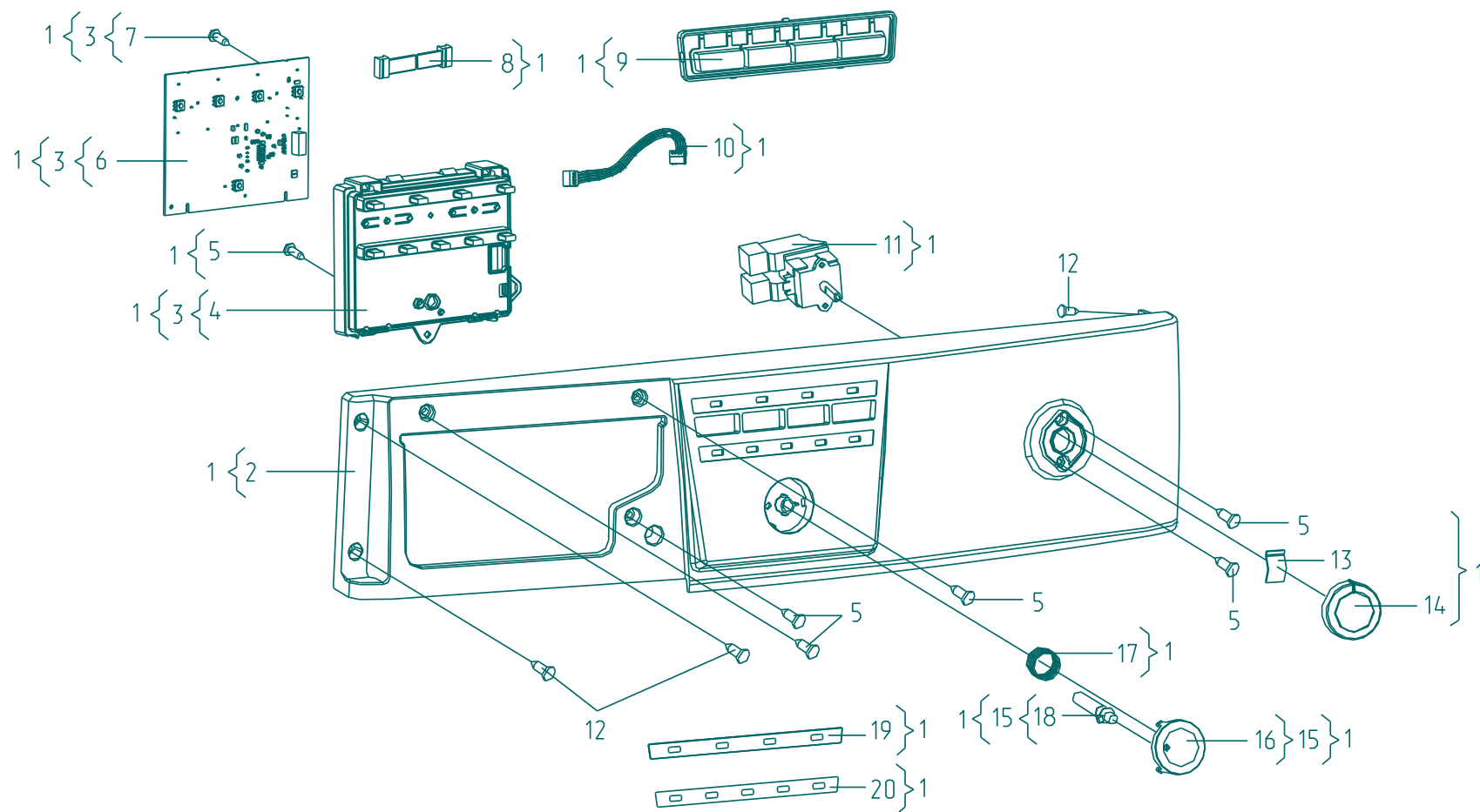
Рисунок 2 - Панель управления
