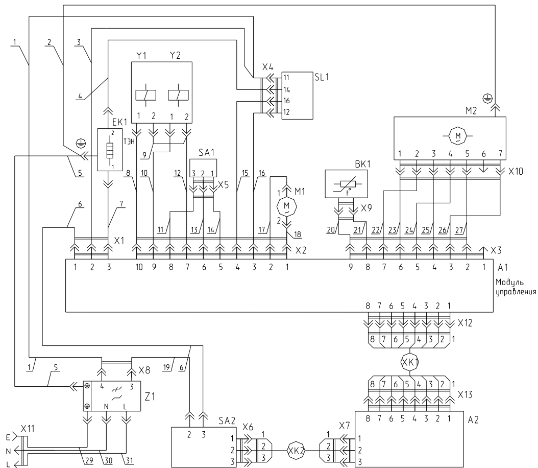
Рисунок А.1 - Схема электрическая принципиальная и соединений машин СМА 35М101-XXX, СМА 35М81-XXX, СМА 45У101-XXX, СМА 45У81-XXX, СМА 50С101-XXX, СМА 50С121-XXX, СМА 50С81-XXX, СМА 60К81-XXX, СМА 60К101-XXX
