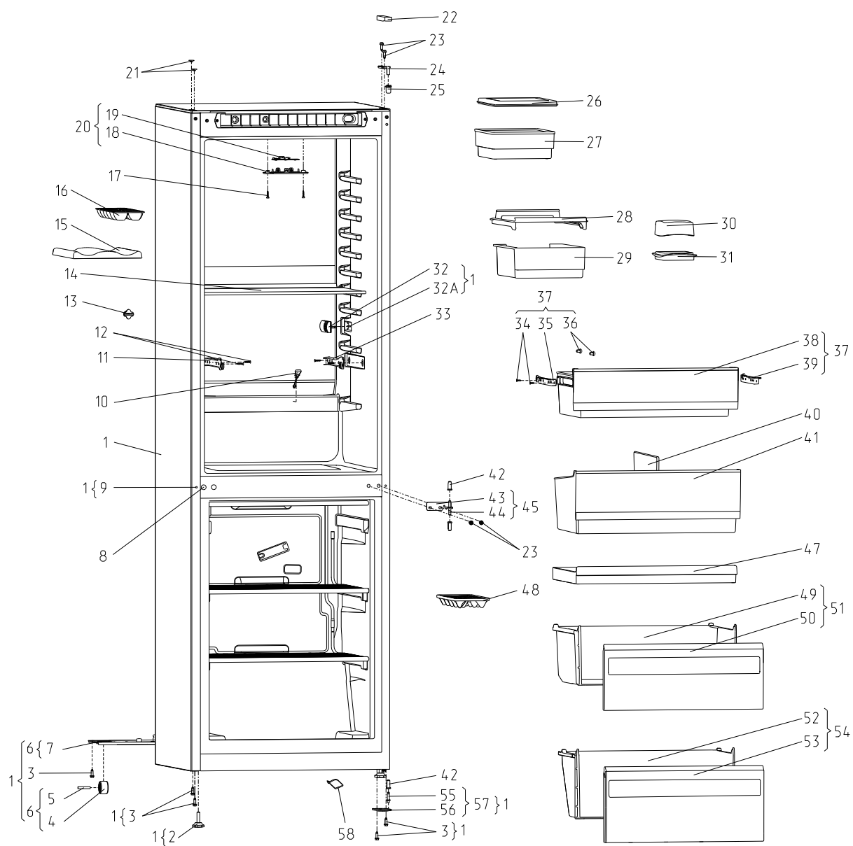
Рисунок 2 - Шкаф
