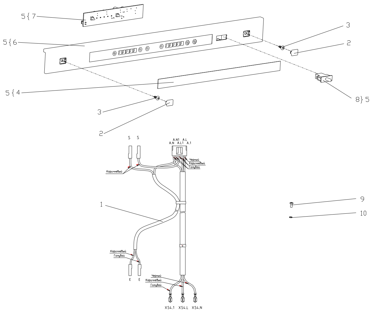
Рисунок 5 - Электропроводка
