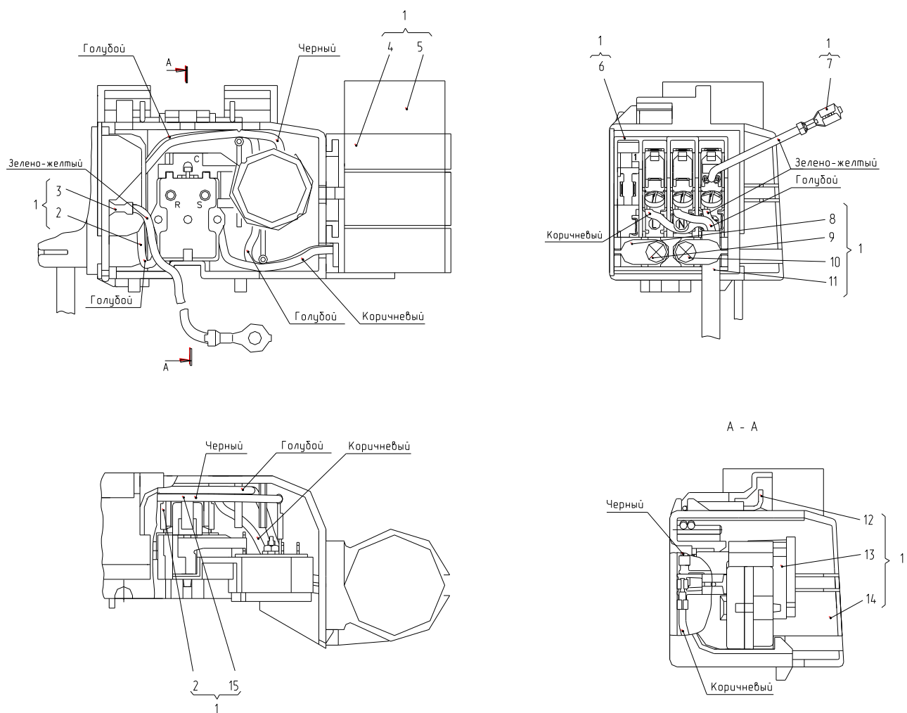
Рисунок 6 - Шнур питания с компрессором типа CTC
