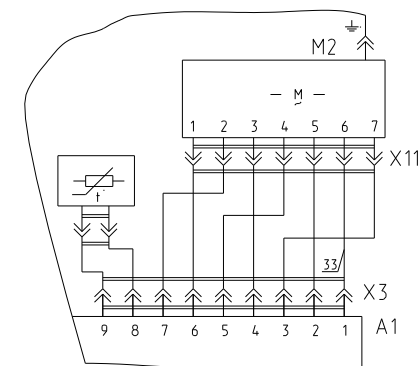
Рисунок А.2 - Схема электрическая принципиальная Остальное см. рисунок А.1
