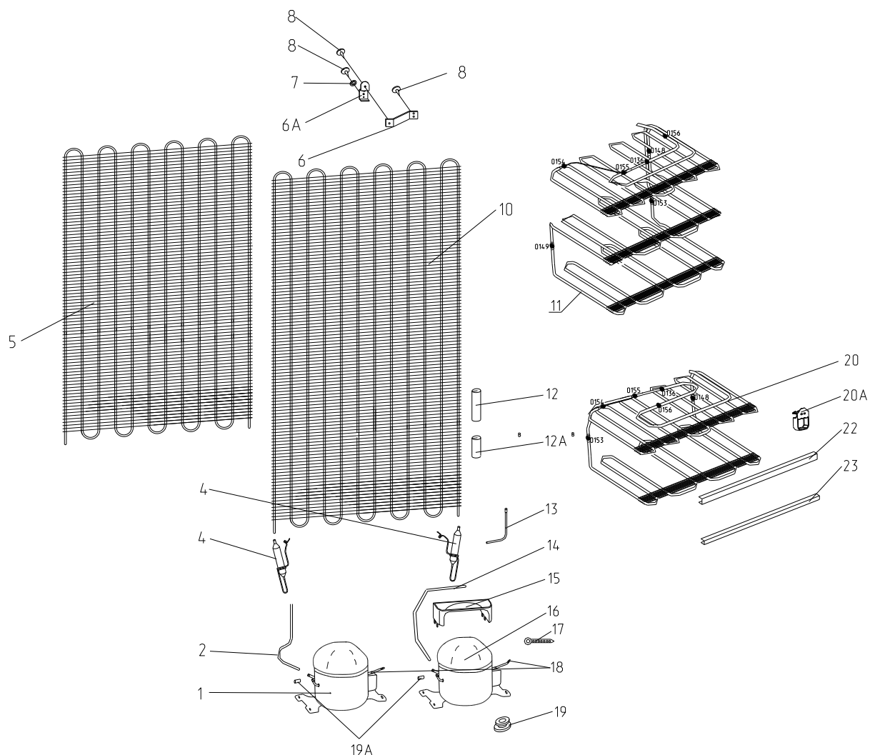
Рисунок 5 - холодильный агрегат
