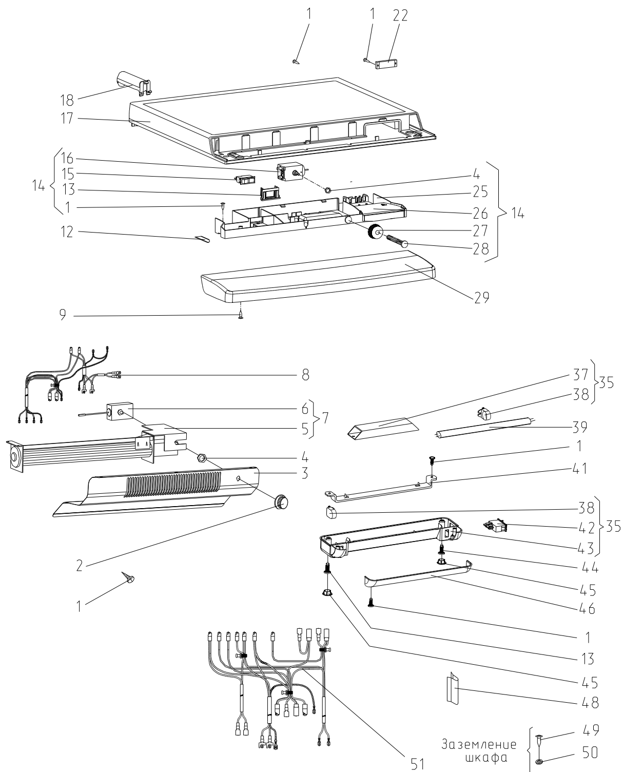
Рисунок 6 - электропроводка
