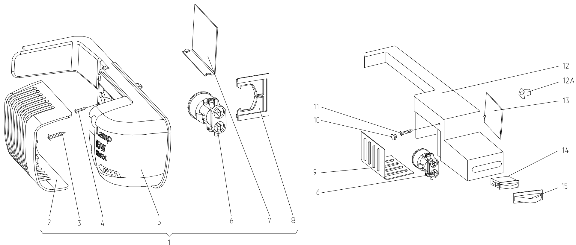
Рисунок 6 - Панель монтажная
