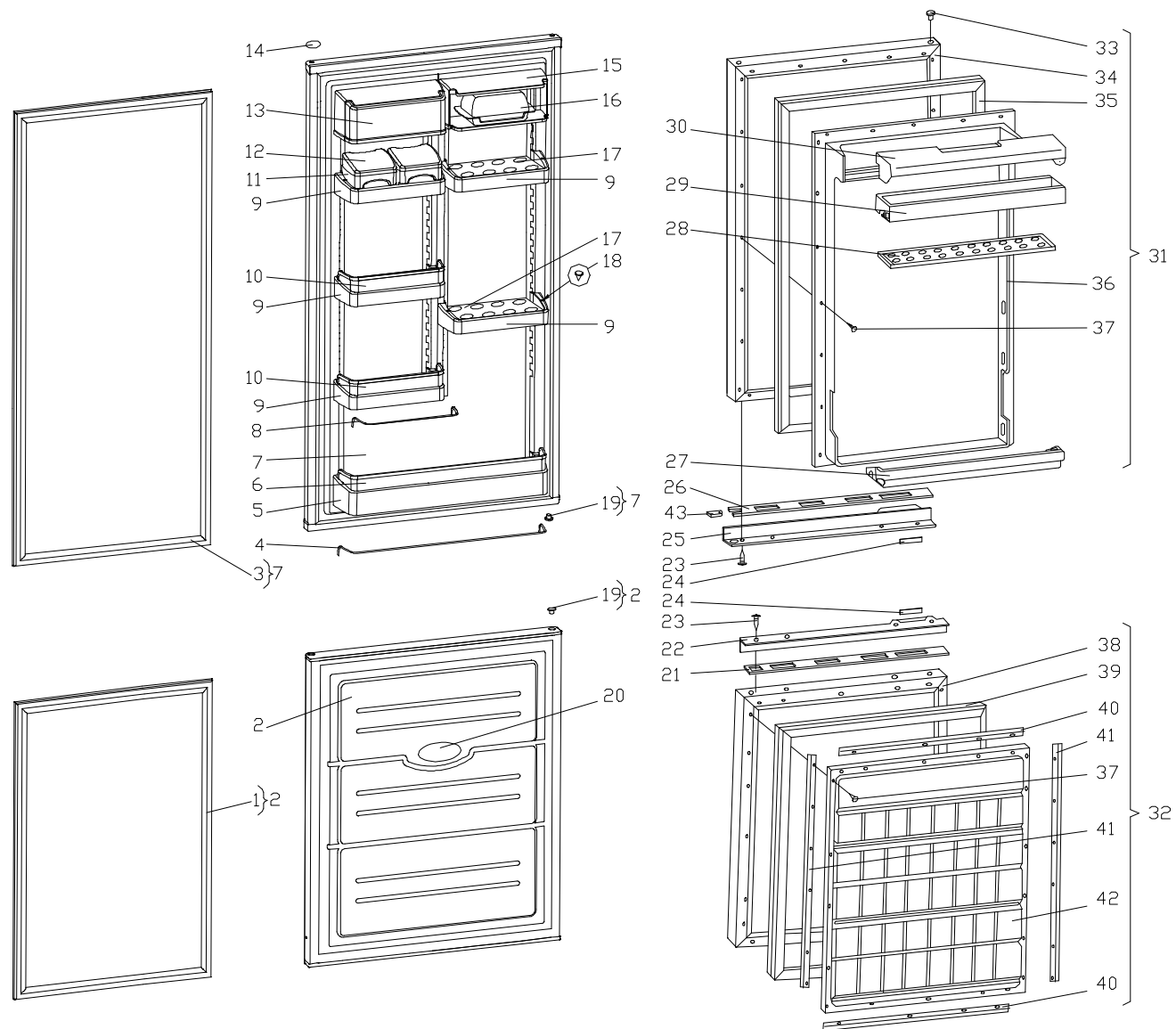
Рисунок 3 - Двери
