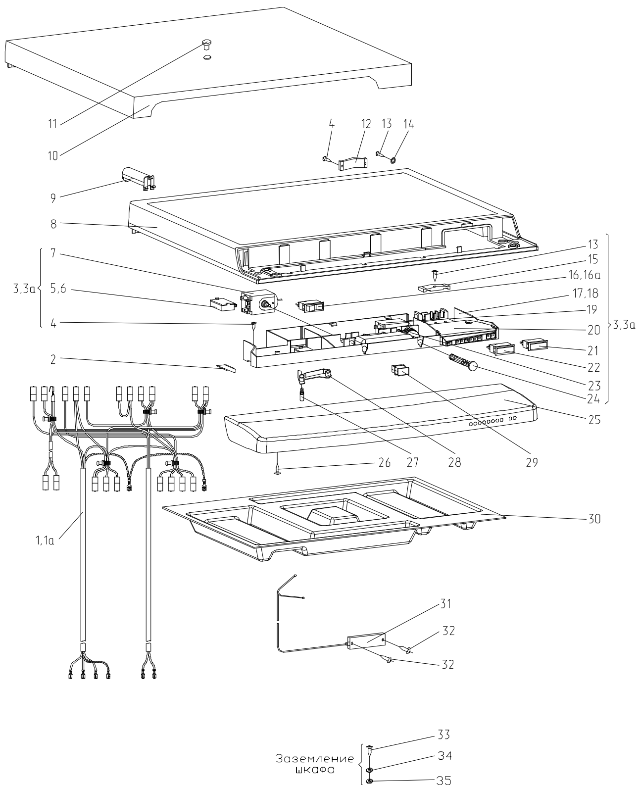
Рисунок 5 - Электропроводка
