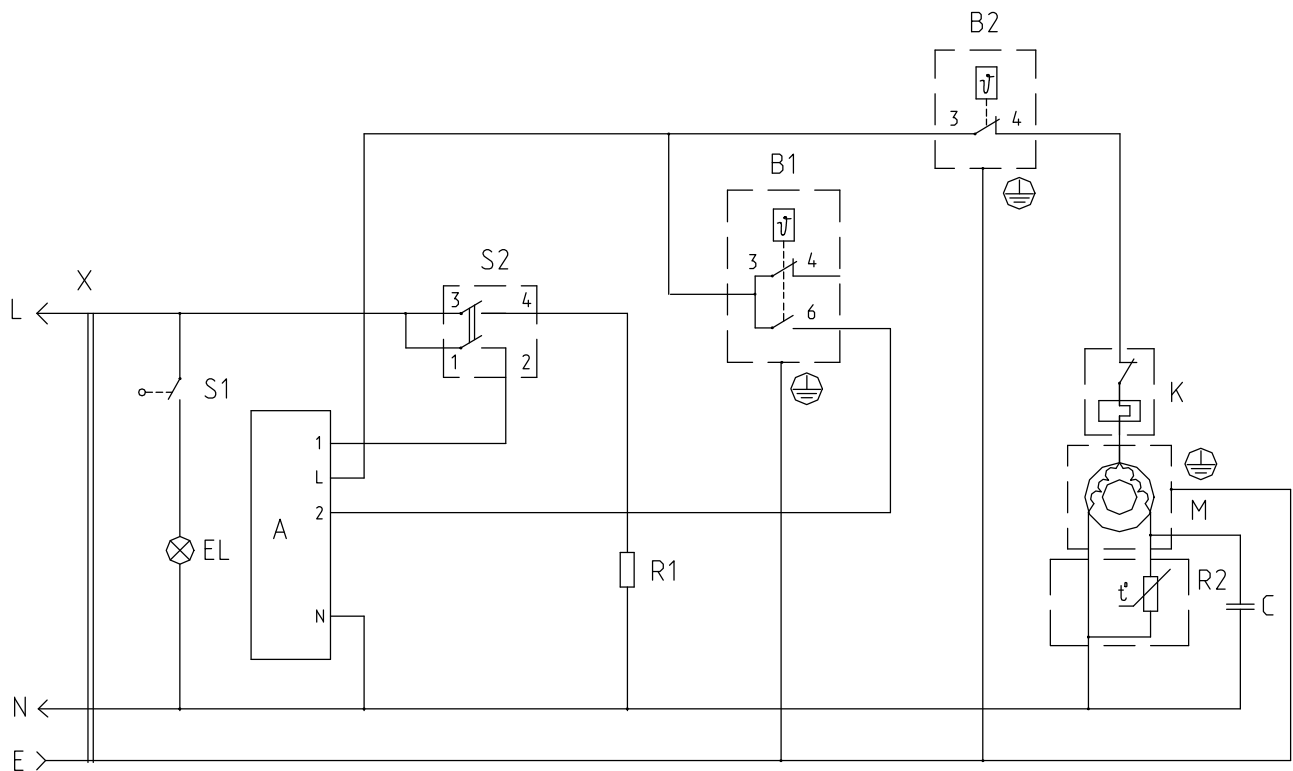
Рисунок А.5 – Схема электрическая принципиальная холодильников КШД-151,КШД-152,МХМ-161, МХМ-162,МХМ-160,МХМ161-50,МХМ-162-50
