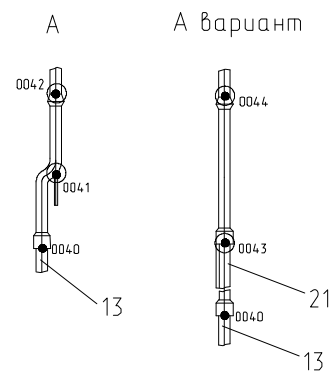
Рисунок 4 - Схема холодильного агрегата
