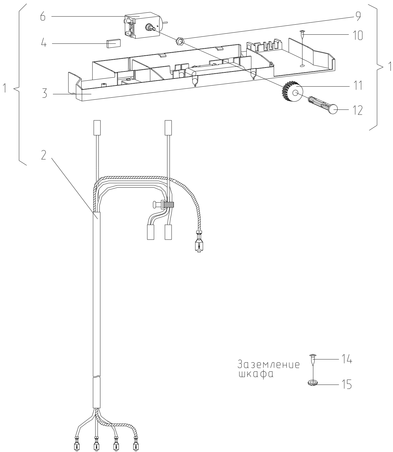
Рисунок 6 - Электропроводка
