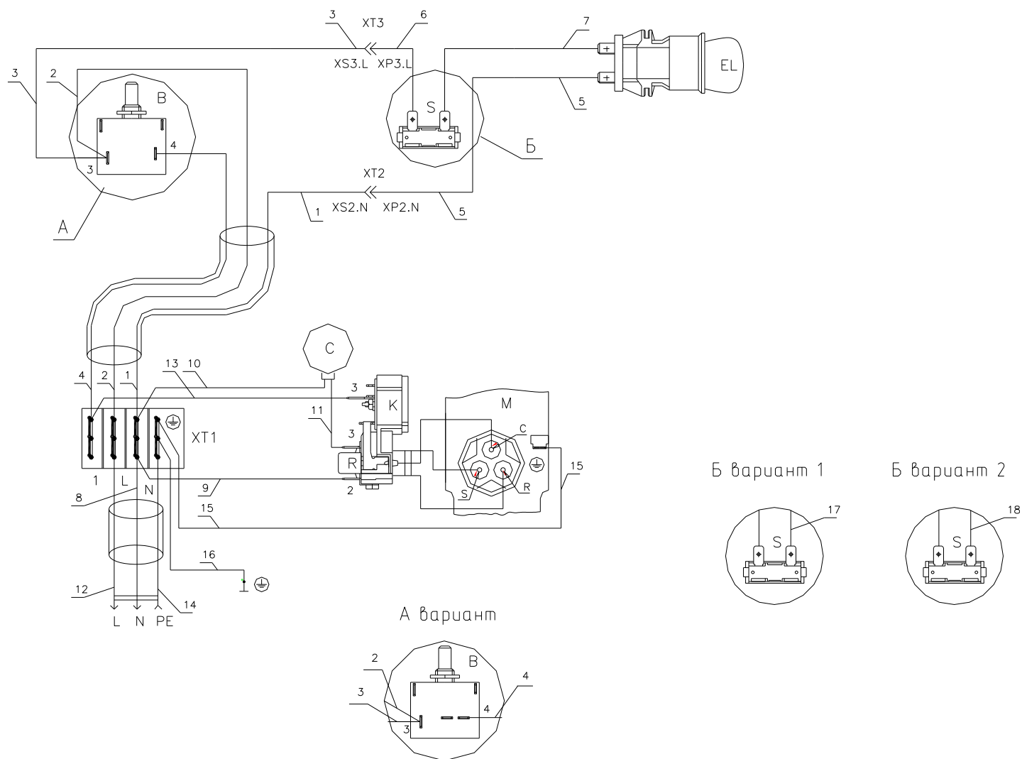
Соединения проводов указаны в таблице А.2. Рисунок А.2 - Схема электрическая соединений
