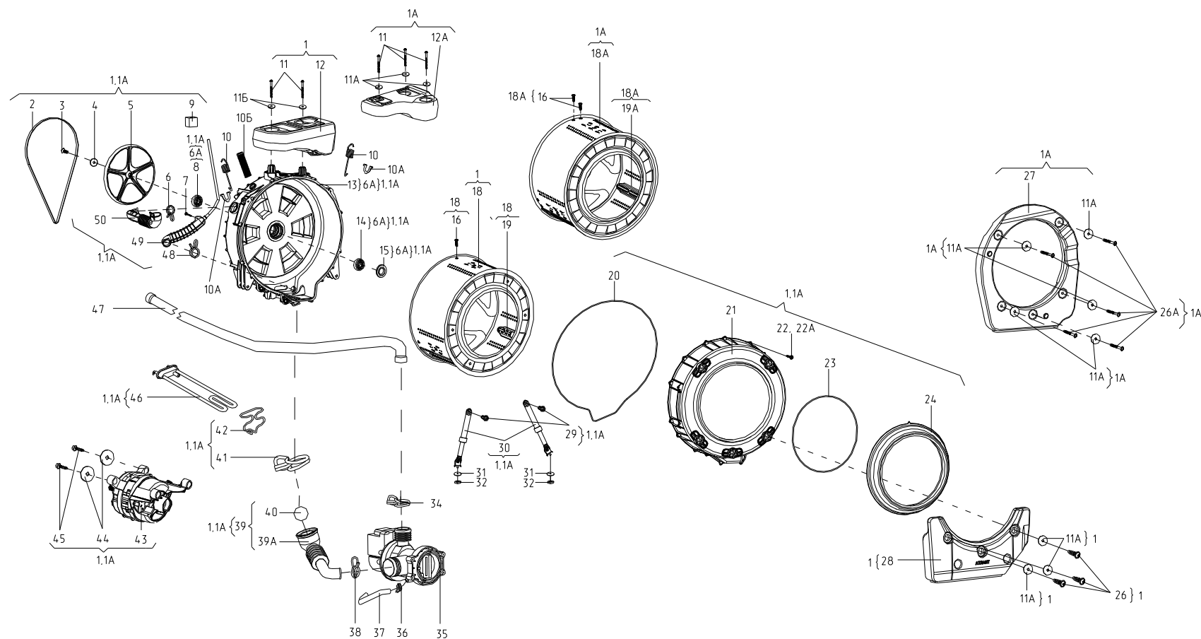
Рисунок 4 - Колебательная система
