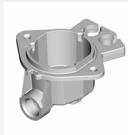
86 Корпус горелки полубыстрого действия 345004131000, 600080015
