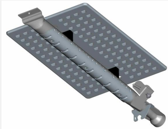
1 Горелка жарочная 1100.23.0.000-04
