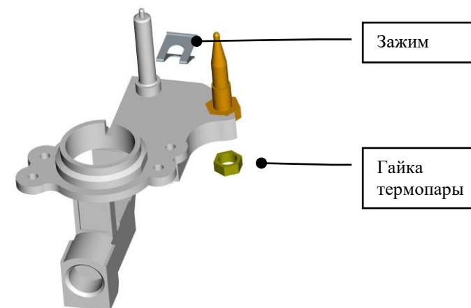
Корпус горелки повышенной мощности
