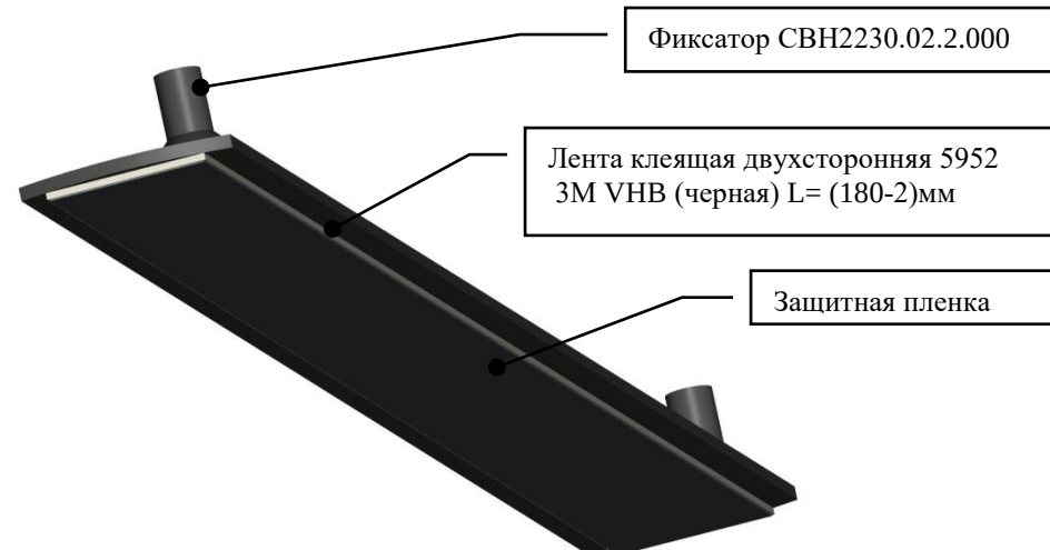
Фиксатор с двухсторонним скотчем СВН2230.02.3.000
