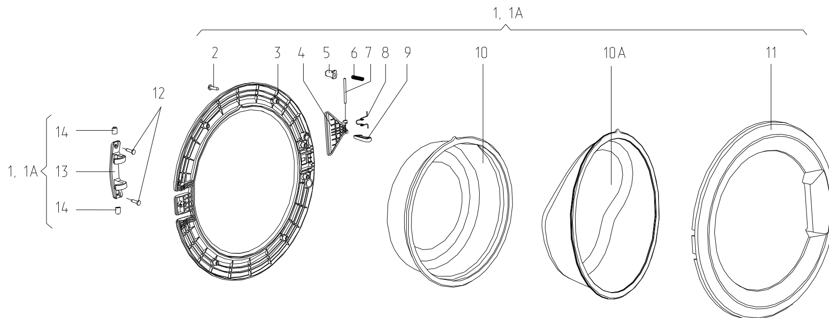
Рисунок 5 - Дверца
