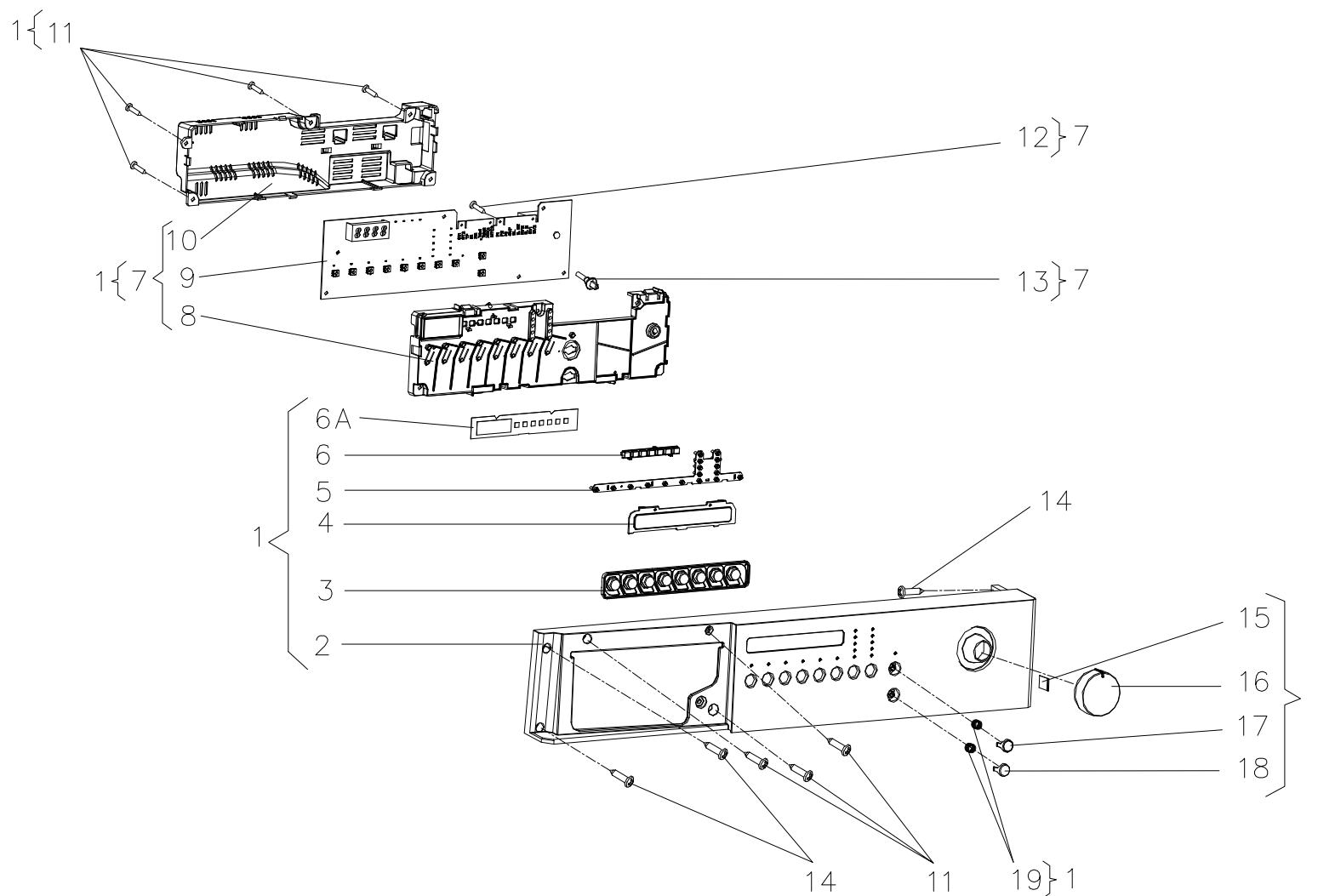
Рисунок 2 - Панель управления
