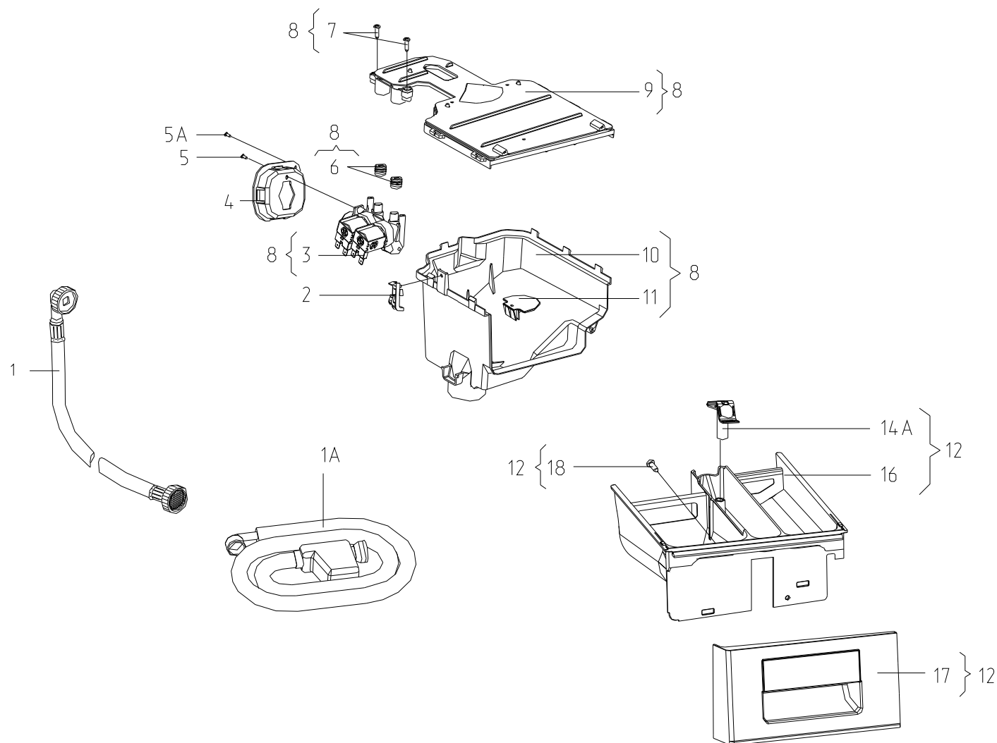
Рисунок 3 - Система налива воды
