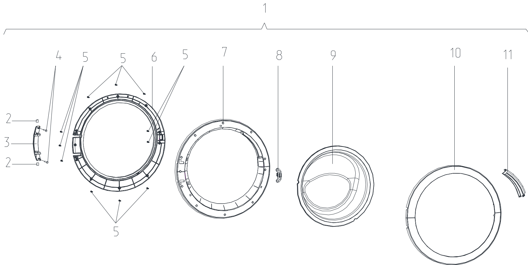
Рисунок 5 - Дверца
