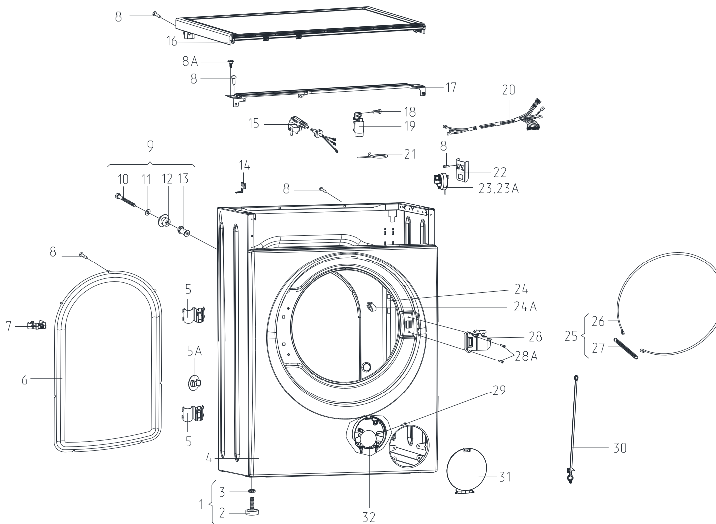
Рисунок 1 - Корпус
