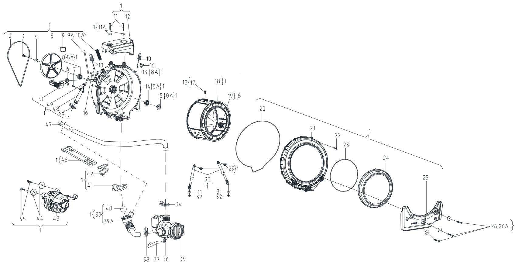
Рисунок 4 - Колебательная система
