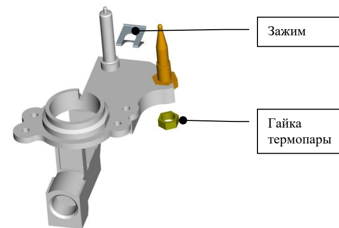
Корпус горелки повышенной мощности
