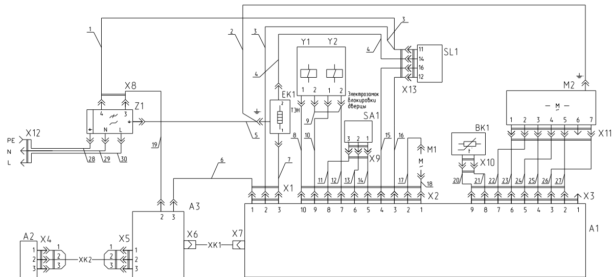
Рисунок А.1 – Схема электрическая принципиальная и соединений
