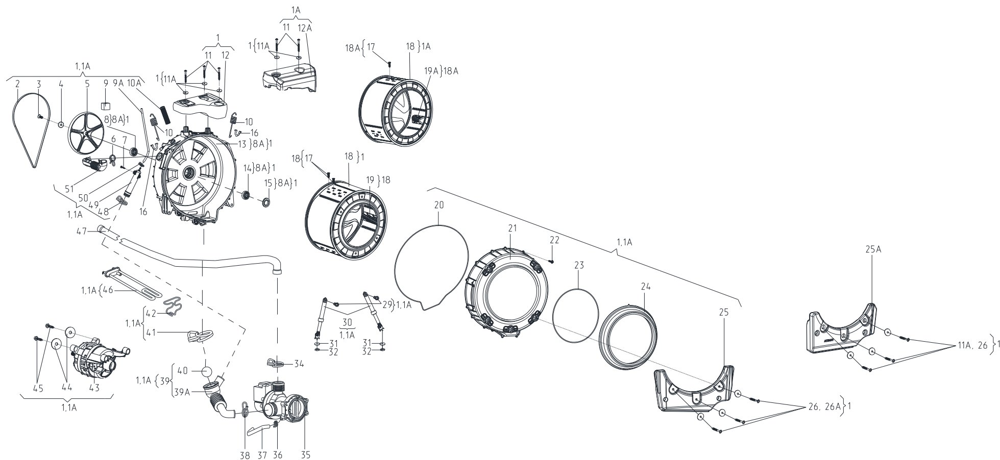
Рисунок 4 - Колебательная система
