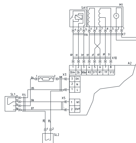
Рисунок А.4- Схема электрическая принципиальная и соединений СМА 60У1210-А-XX, СМА 70С1410-А-XX
