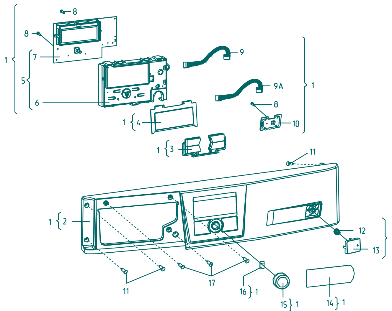
Рисунок 2 - Панель управления
