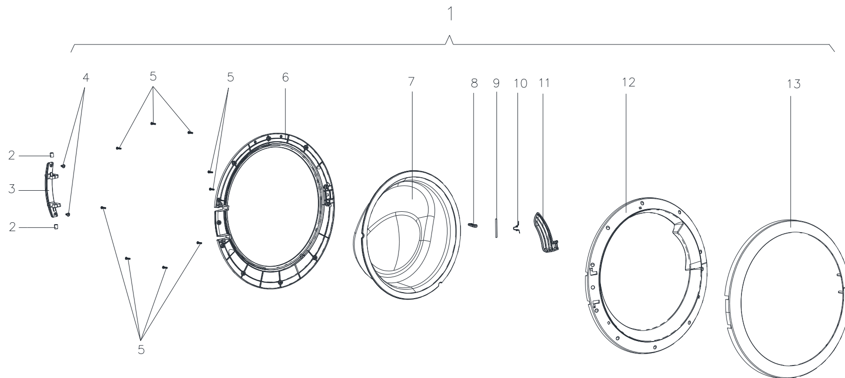
Рисунок 5 - Дверца
