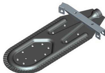
Горелка духовки
